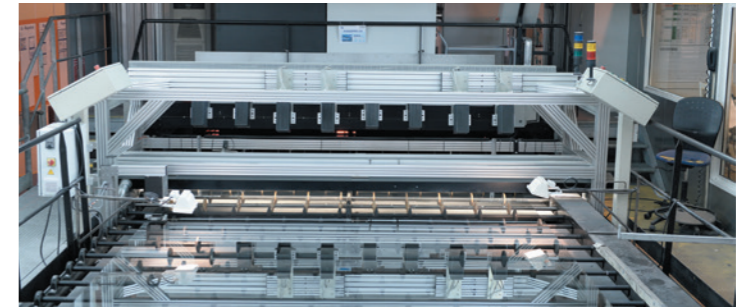
Magnetron-Fertigungslinie
